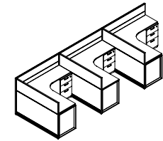
名称 Name 屏风 型号 Model BG-P015 尺寸 Size 1400W*4200D*1200H
