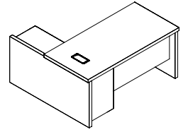
名称 Name 班台 型号 Model BG-6218 尺寸 Size 1600W*1400D*760H 1800W*1600D*750H
