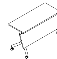
名称 Name 条桌 型号 Model BG-P023 尺寸 Size 1200W*400D*750
