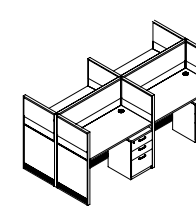
名称 Name 屏风 型号 Model BG-P013 尺寸 Size 2400W*1200D*1200H
