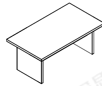
名称 Name 班台 型号 Model BG-6210 尺寸 Size 1800W*900D*750H 2000W*1000D*750H 2400W*1200D*750H
