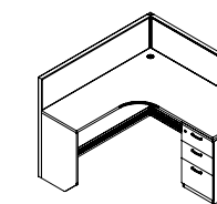
名称 Name 屏风 型号 Model BG-P017 尺寸 Size 1200W*1400D*1200H
