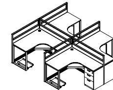
名称 Name 屏风 型号 Model BG-P019 尺寸 Size 2800W*2800D*1200H
