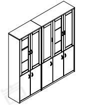
名称 Name 文件柜 型号 Model BG-6250 尺寸 Size 2000W*400D*2000H
