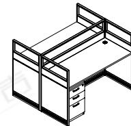
名称 Name 屏风 型号 Model BG-P014 尺寸 Size 1400W*1200D*1200H
