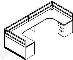
名称 Name 屏风 型号 Model BG-P018 尺寸 Size 3000W*1400D*1200H
